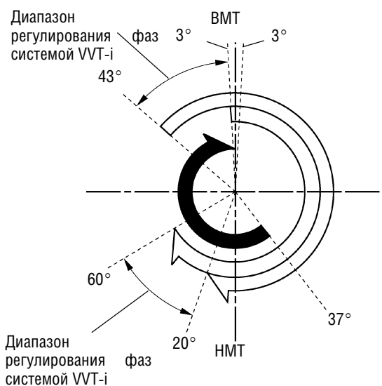
ДВИГАТЕЛЬ 1AZ-FE
