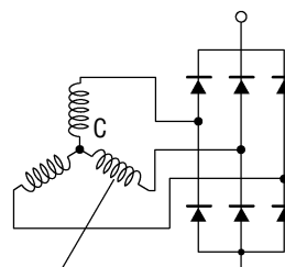
Трехфазная обмотка
