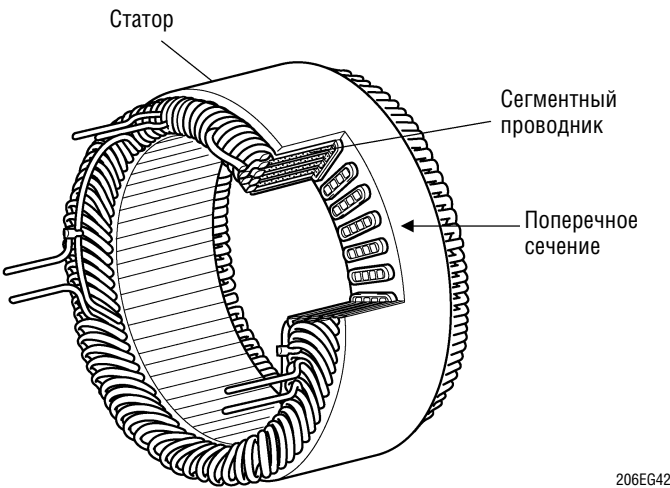
Статор сегментного генератора
