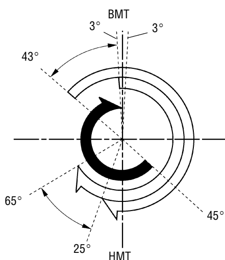
ДВИГАТЕЛЬ 2AZ-FE
