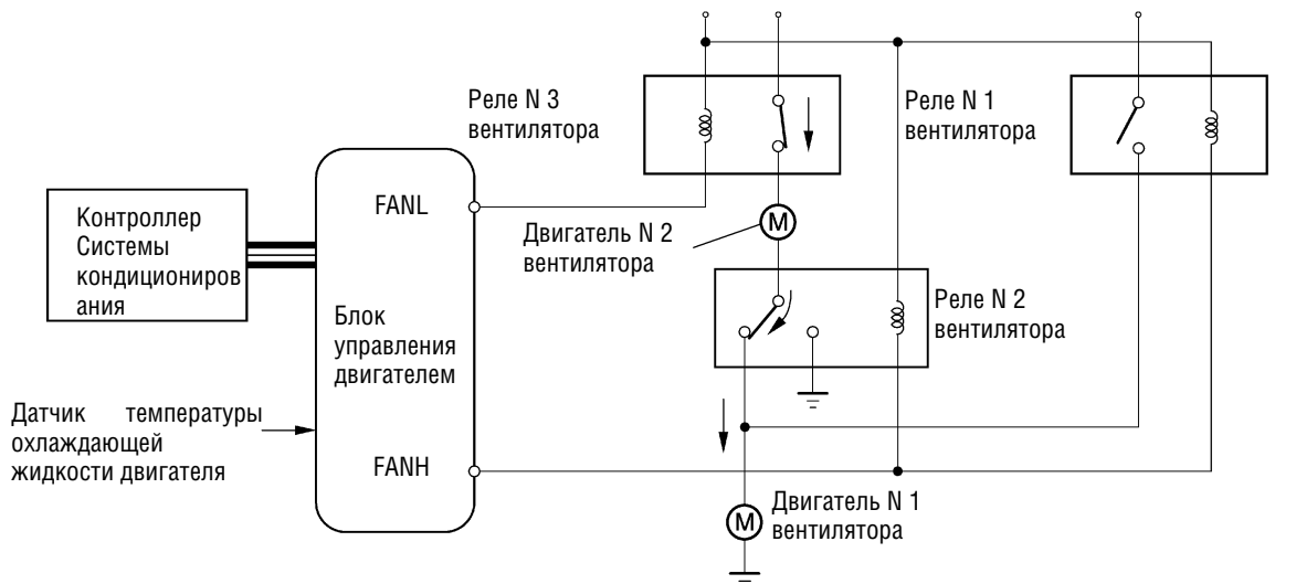
Низкая скорость вращения (последовательное соединение)
