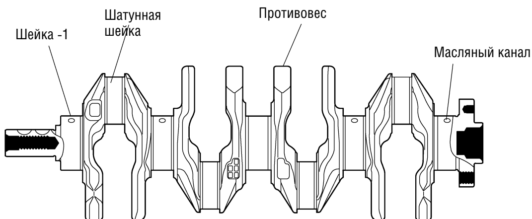
ДВИГАТЕЛЬ 1AZ-FE
