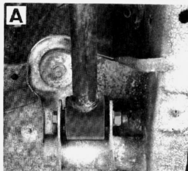
Desmontaje de un tirante longitudinal
