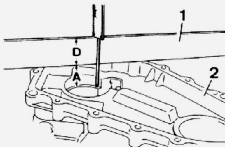
Medición del juego de los rodamientos 1. Regla - 2. Cárter trasero 3. Cárter delantero.
