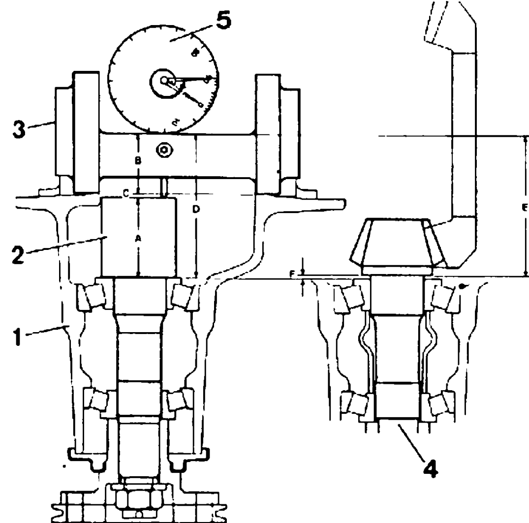
Reglaje de la distancia cónica.
