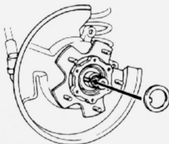
Montaje de la arandela de pestaña.
