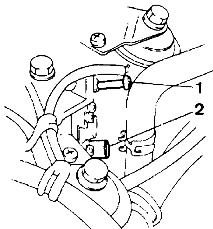
Reglaje del ralenti 1. Tornillo de régimen - 2. Tornillo de riqueza.
