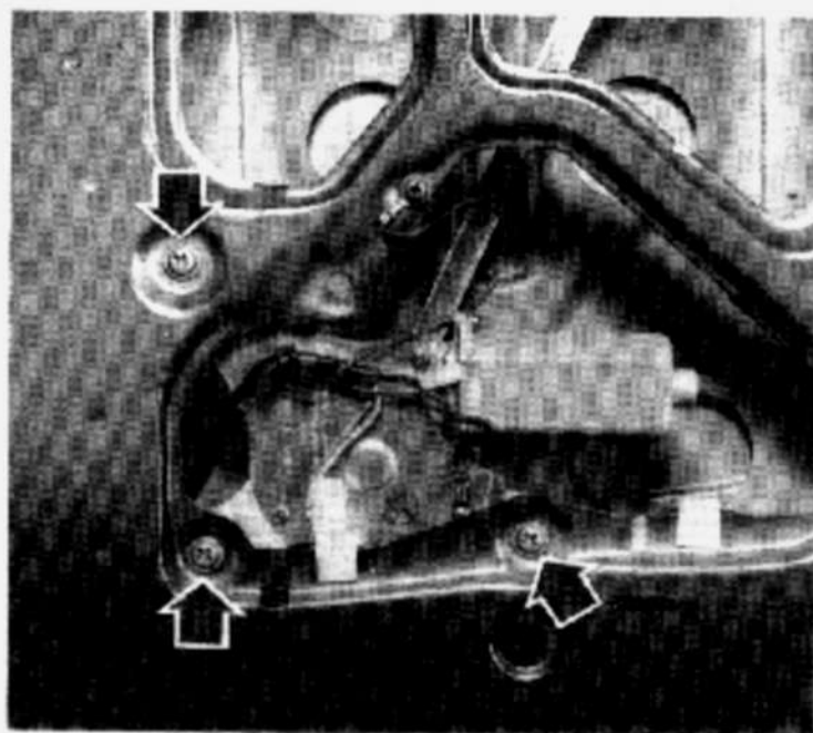
Fijación del mecanismo de limpiaventa trasera.
