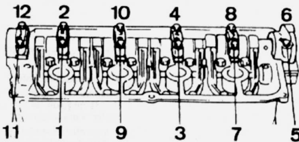
Orden de aflojamiento de tapas de cojinete de árbol de levas.
