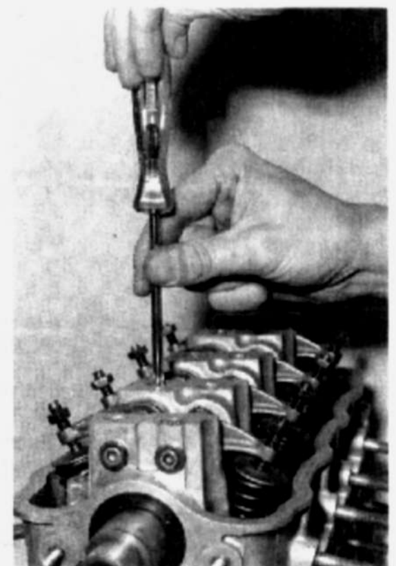
Desmontaje de los tornillos de sujeción de los ejes de balancines.
