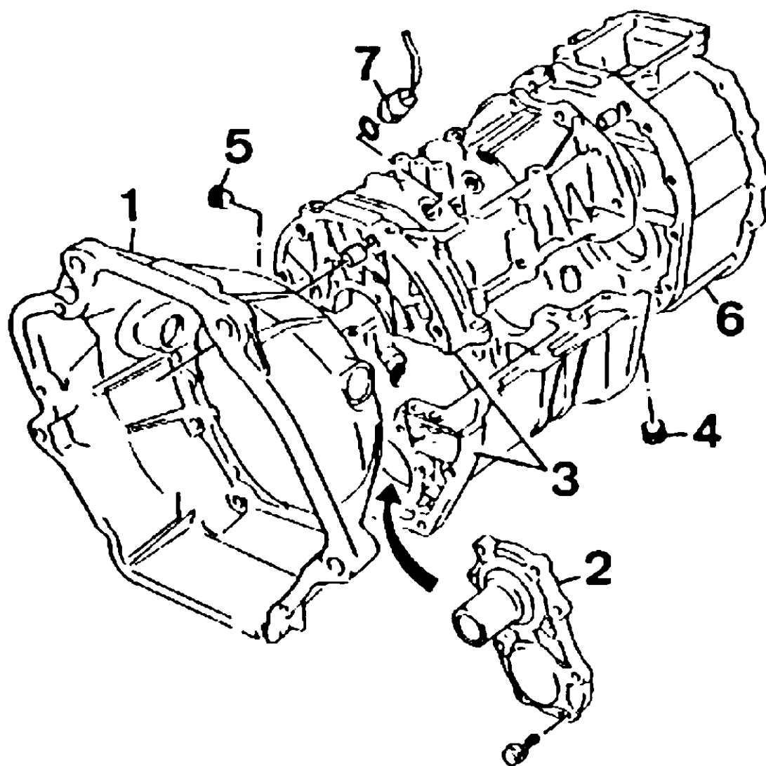
1. Cárter de embrague - 2. Brida de rodamiento y guía del cojinete de empuje - 3. Cárter de pinonería - 4. Tapón de vaciado - 5. Tapon de llenado y nivel - 6. Cárter trasero - 7. Contactor de luces de marcha atrás.
