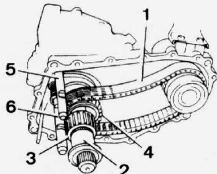
Desarmado de la caja de reenvío. 1. Cadena - 2. Casquillo de rodamiento - 3. Rodamiento de agujas - 4. Piñón - 5. Eje de horquilla de marchas cortas o largas - 6. Eje de horquilla de cuatro ruedas motrices.
