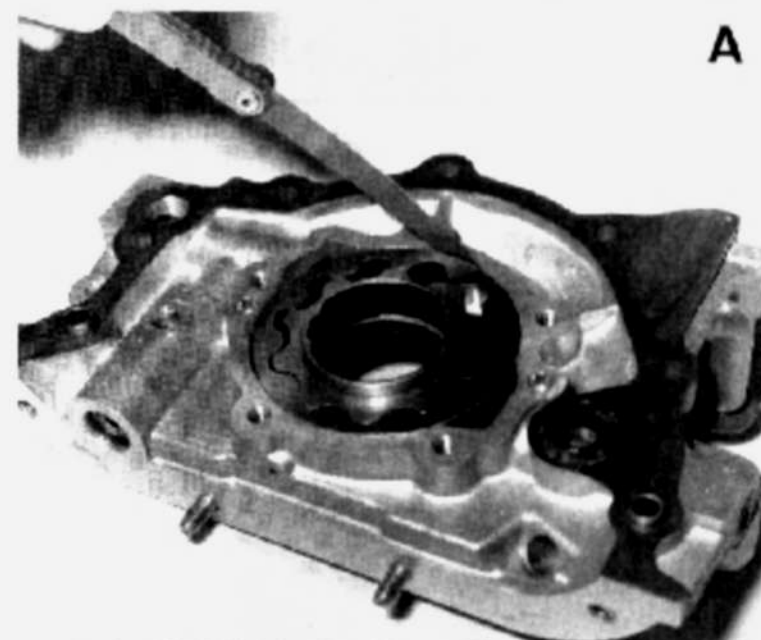
Control de los juegos de bomba de aceite A. Radial - B. Axial.
