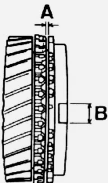
Control de los sincronizadores. A. Juego entre anillo y piñón B. Ancho de las muescas de las chavetas.
