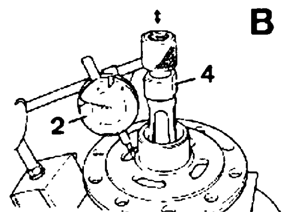
Medición del juego axial de los planetarios
