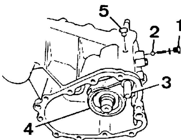
Desmontaje del eje de cambio de gama. 1. Tapon - 2. Bola - 3. Eje de horquilla - 4. Desplazable - 5. Tapón de plástico.
