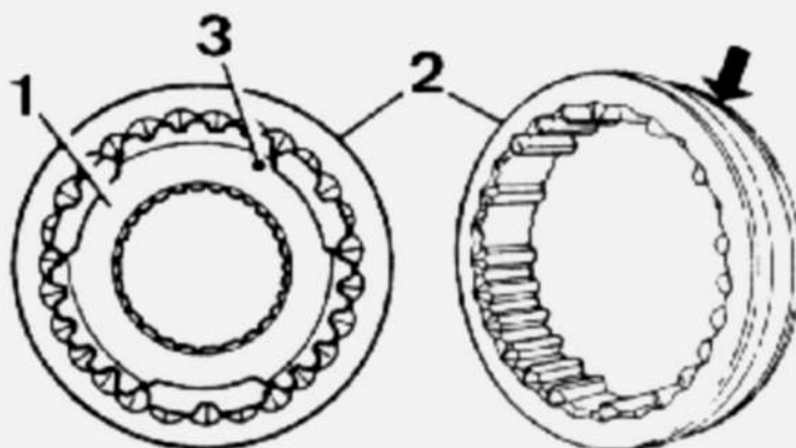
Ensamblado del cubo de garras de cambio a cuatro ruedas motrices. 1. Cubo - 2. Desplazable 3. Punzonado - Flecha: ranura.
