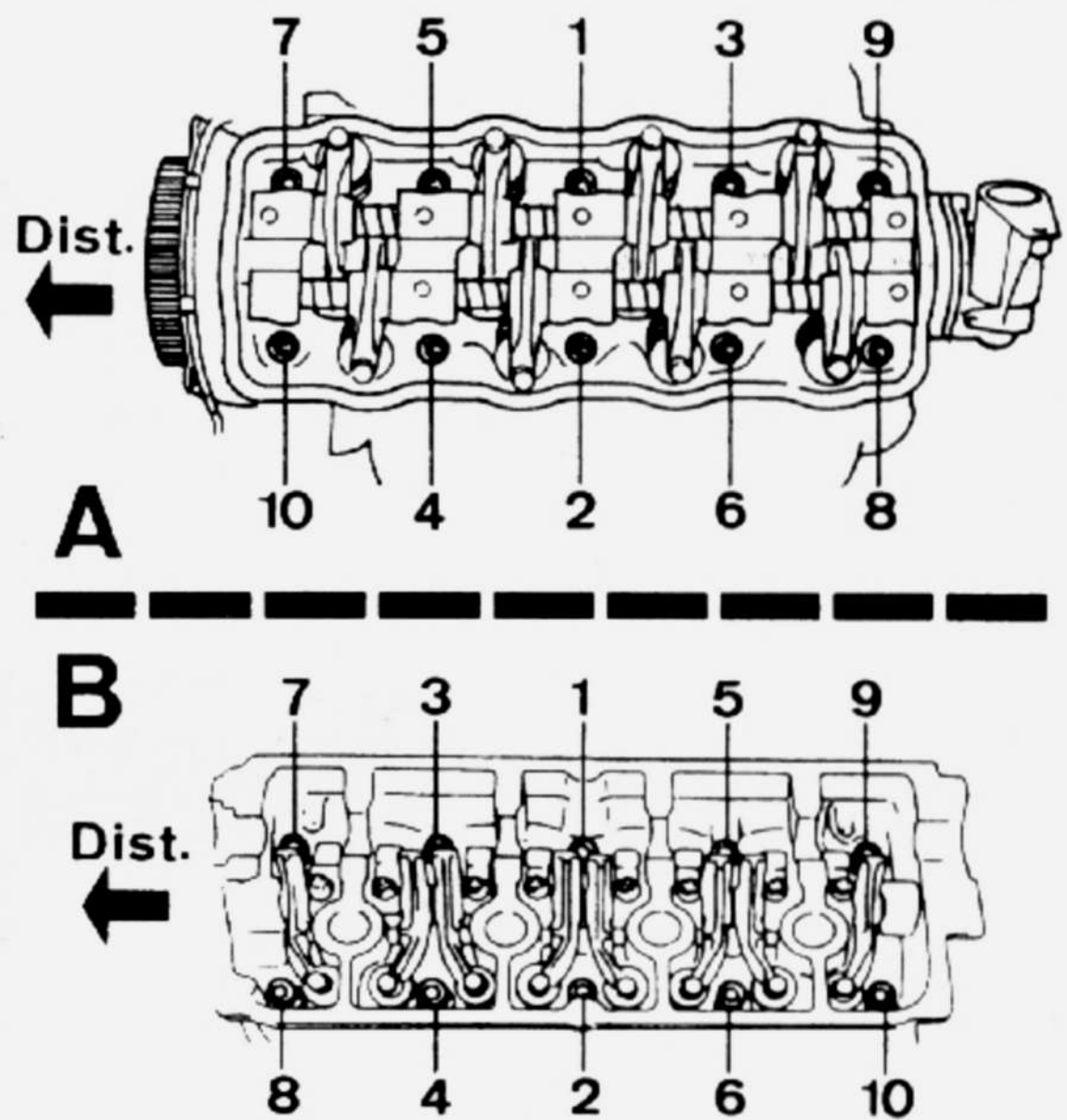
Orden de apriete de la culata. A. Motores de 8 válvulas - B. Motores de 16 válvulas.
