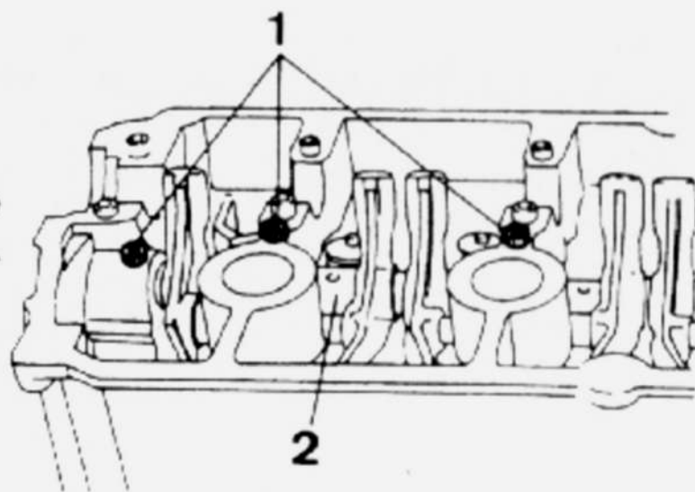
Desmontaje del eje de balancines 1. Tornillo de fijación - 2. Eje.
