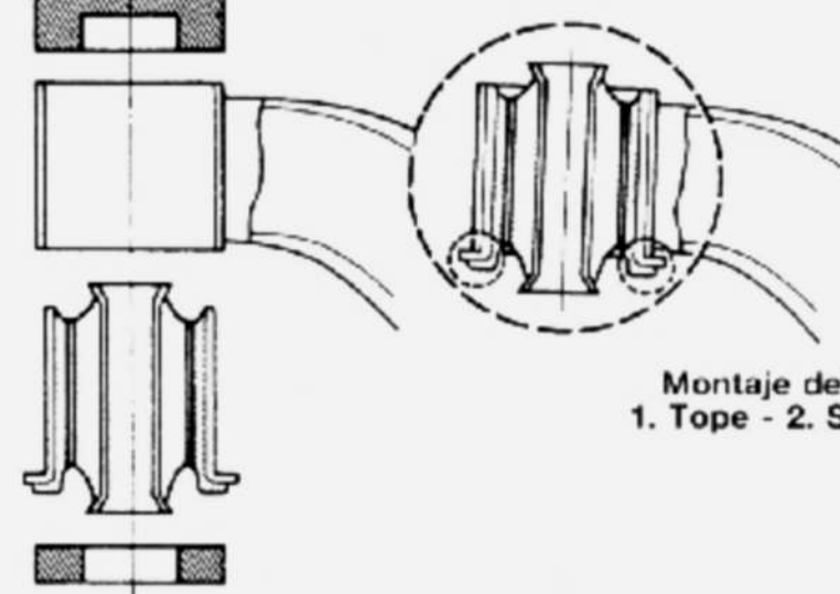
Recorte del collarín del silentbloc delantero.
