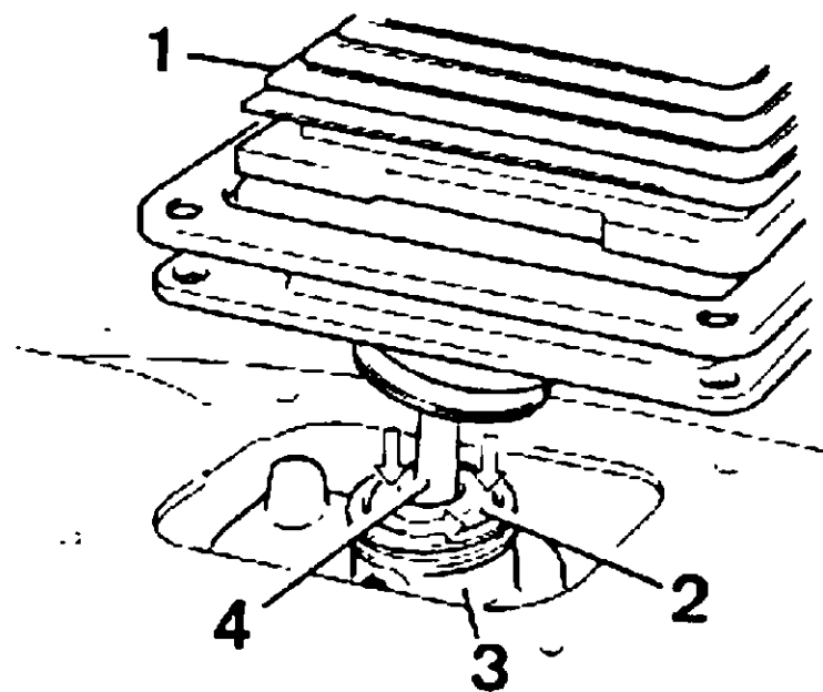
Desmontaje de la palanca de mando. 1. Fuelle protector - 2. Tapa del cárter - 3. Cárter de la palanca - 4. Palanca.
