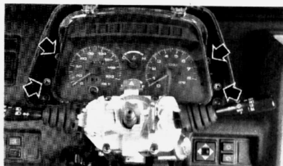
Tornillos de fijación del cuadro de instrumentos.
