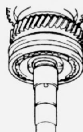
Ensamblado del eje secundario. 1. Piñón de 5ª - 2. Arandela de tope (dirigir las ranuras de engrase hacia el piñón).
