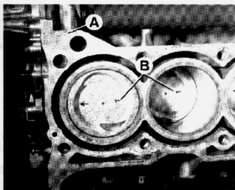
Montaje de los pistones A. Marcas del diámetro de cilindros - B. Marcas de emparejamiento de pistones (las mismas que las del plano del cárter). Las flechas de los pistones van dirigidas hacia la distribución.
