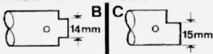
Marcas de los ejes de balancines
