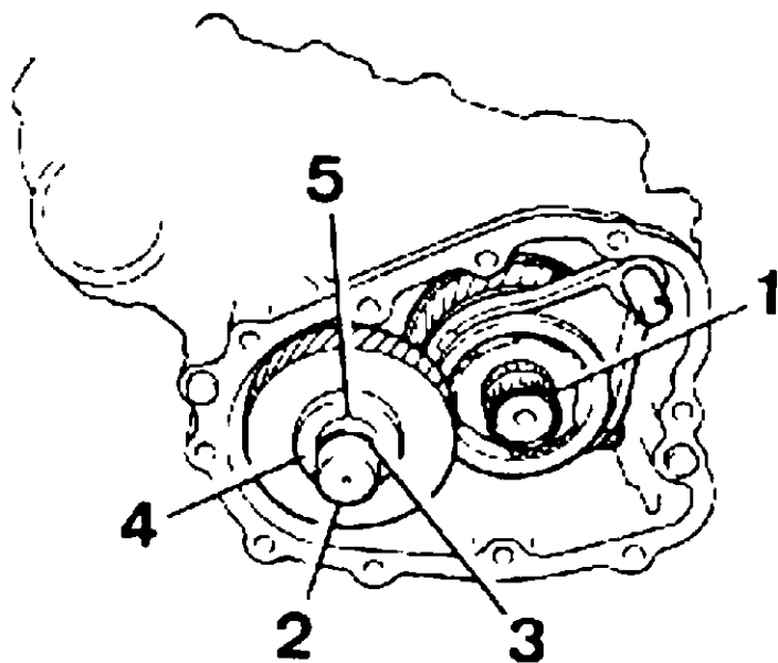
Desarmado de la caja de reenvío. 1. Rodamiento de agujas de guía del eje primario 2. Eje intermedio - 3. Junta tórica - 4. Arandela de tope - 5. Bola de bloqueo.
