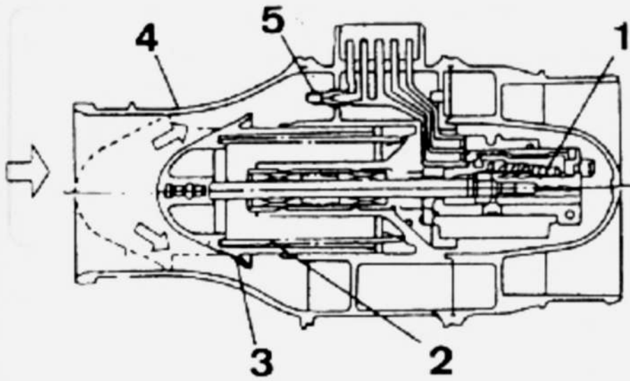
Corte del caudalímetro
