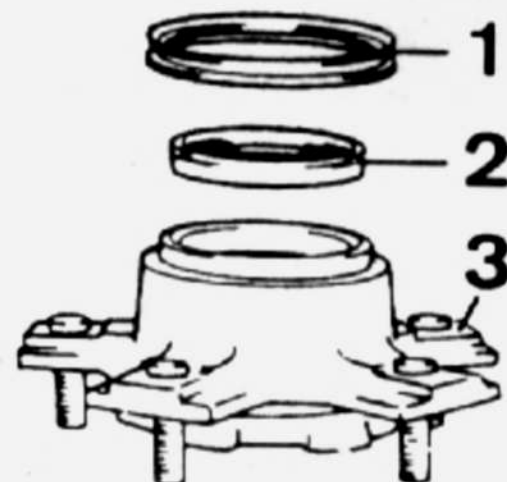
Montaje de los retenes 1. Anillo de cierre - 2. Retén interior 3. Cubo.
