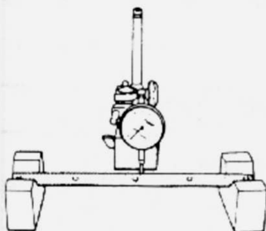
Control del salto del eje de balancines.
