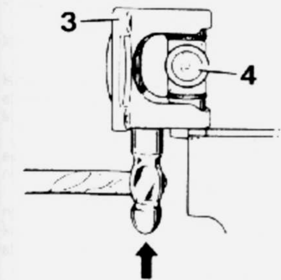
Desarmado de un cardán. 1. Herramientas especiales - 2. Rodamiento - 3. Cardán - 4. Cruceta.
