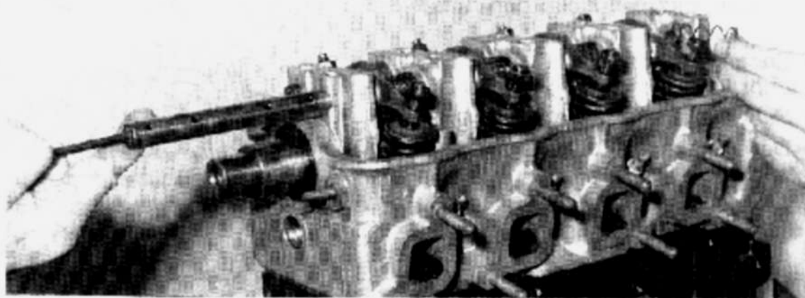
Desmontaje de un eje de balancines.
