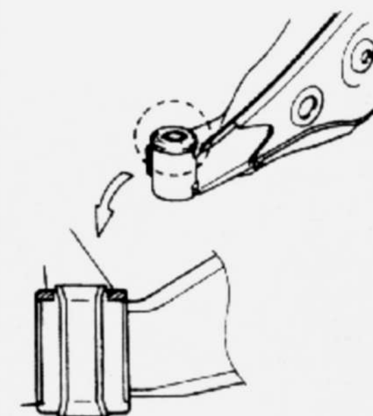
Recorte del collarín del silentbloc trasero 1. Parte a recortar.
