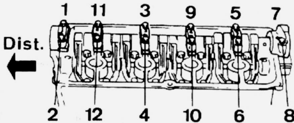
Orden de apriete de las tapas de cojinete de árbol de levas.
