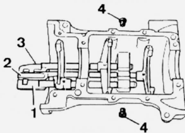
Ensamblado de los ejes de horquillas. 1. Eje de 5ª-marcha atrás - 2. Eje de 3ª-4ª - 3. Eje de 1ª-2ª - 4. Tapones de obturación.
