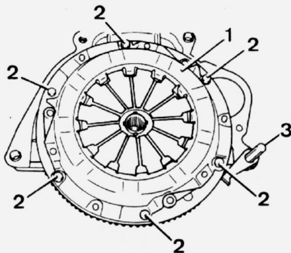
Desmontaje del mecanismo o del disco. 1. Mecanismo - 2. Tornillos de fijación - 3. Herramienta de bloqueo del volante motor.
