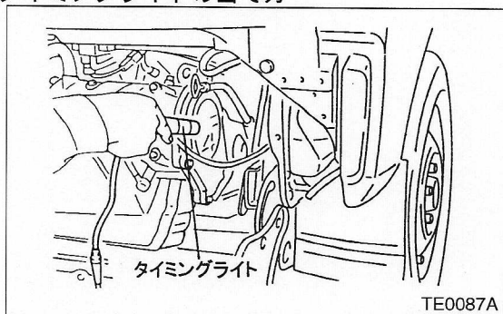
タイミングライトの当て方
