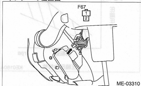
コネクタの位置図
