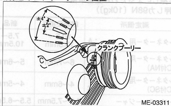
刻線とインジェクターの位置
