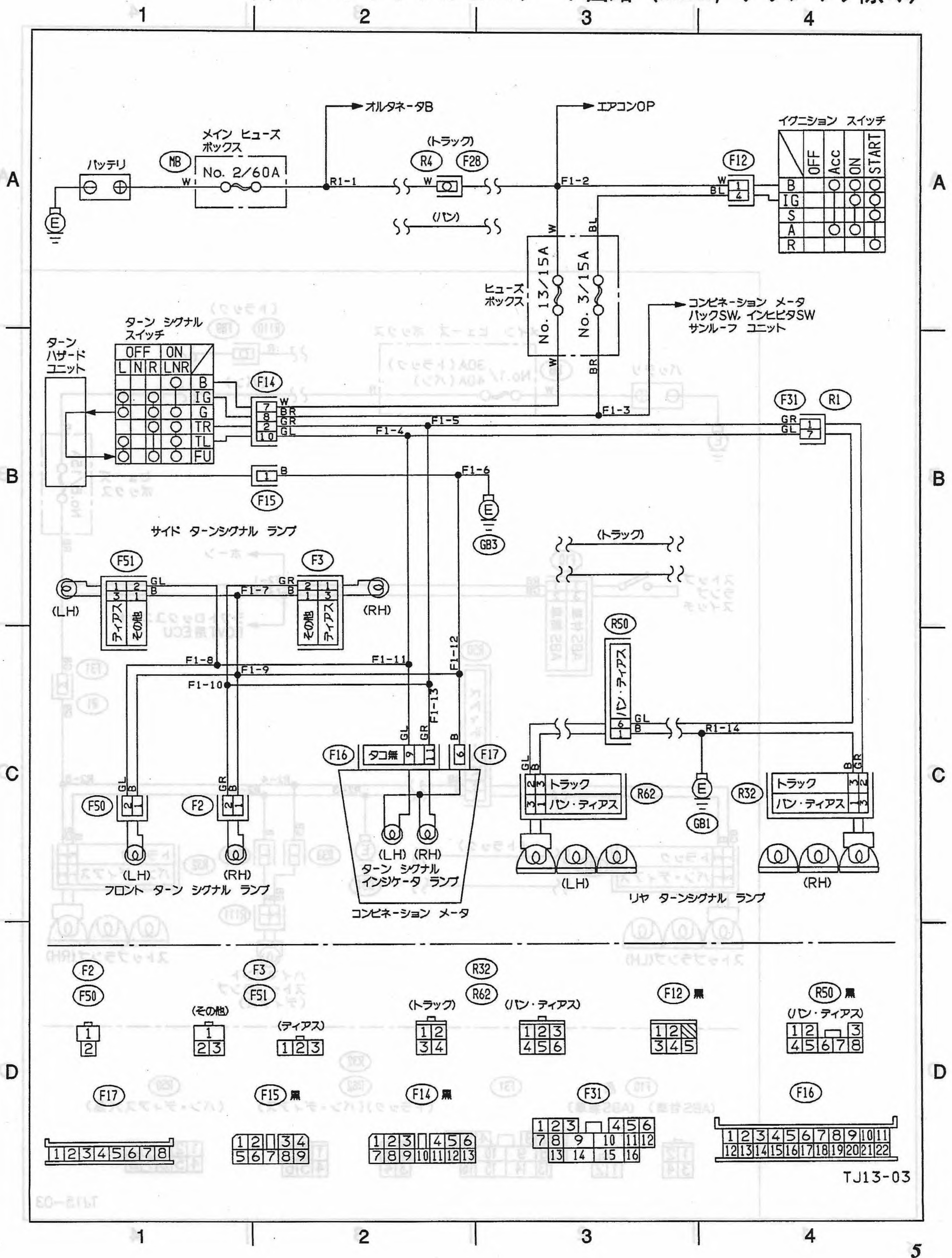
(1) ターンシグナル&ハザード回路 (MSC, クラシック除く)
