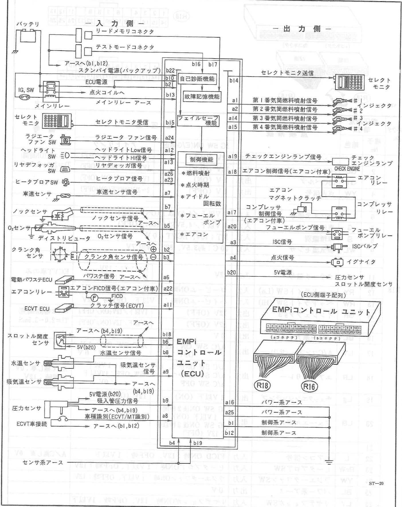
— EMPiシステム入出力図 —
