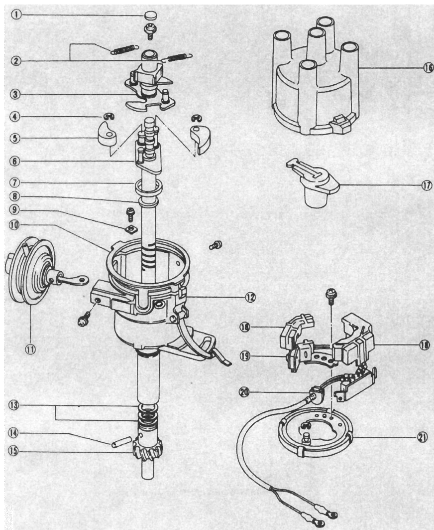
Распределитель Nippondenso модели 100291
