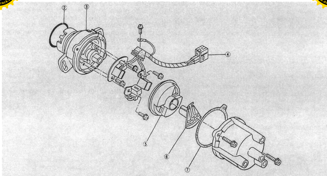
Распределитель Nippondenso модели 100291
