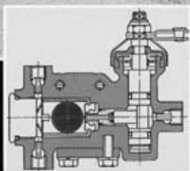
Rückrollbremse „Hill-Holder“
