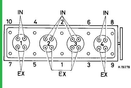
1984 cm³, 16V
