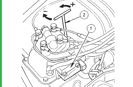
KE-Motronic
