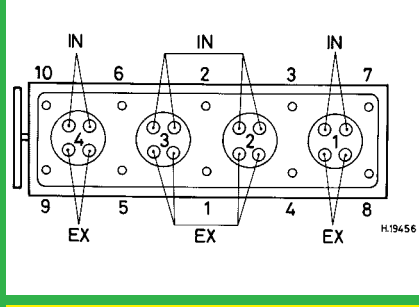
1985 cm 3 , 16V
