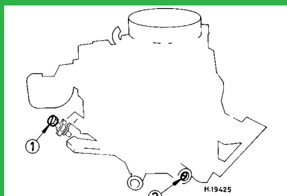
Solex 32 BIS
