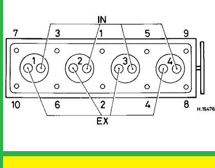
2479 cm³, 8V
