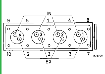
1360 cm³, TU3
