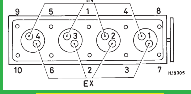
1360 cm³, TU3
