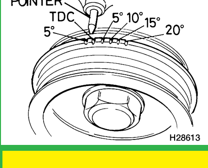
998 cm³, DOHC 16V
