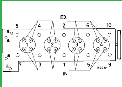
2299 cm 3 , 16V
