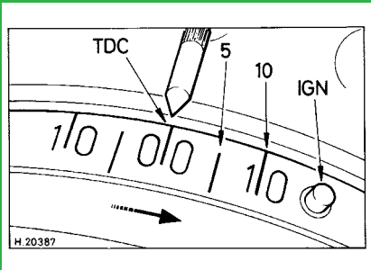
2299 cm 3 , 16V
