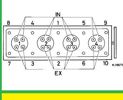
1324 cm³, 16V
