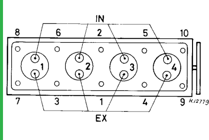
1995 cm³, DOHC 8V
