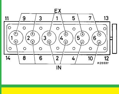
1990 cm³, 12V
