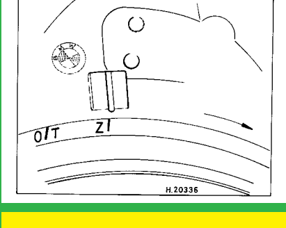
1990 cm³, L-Jetronic
