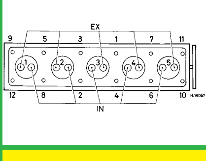
1994 cm³, 10V
