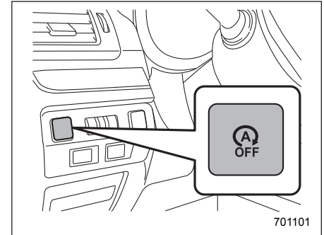
Выключатель системы автоматического запуска/остановки двигателя
