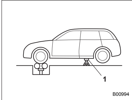
1) Опорная стойка.
